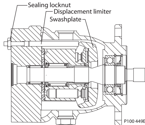
Displacement limiter M35/M44 MV
